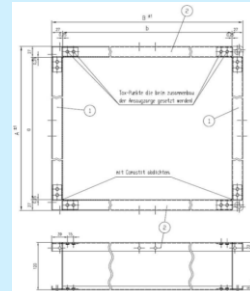
Zarge/connecting piece ZG99 MO25 CN Edelstahl/stainless steel CN Profile in Gehrung geschnitten/mitred profiles Verbindung mit L profilen/connection with L profiles
