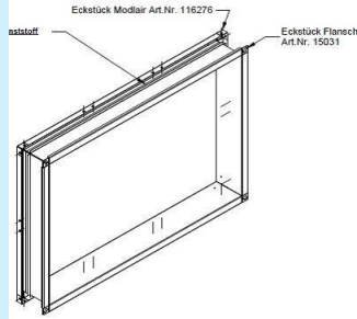
Zarge/connecting piece ZG99 MO25 PB Pulver beschichtet/powder coated PB RAL7035 Verzinkte Eckstücke/galvanized corner pieces
